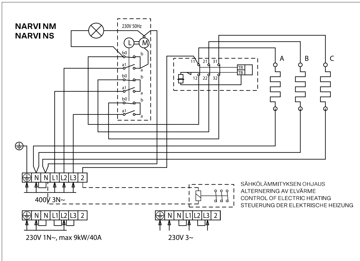
Kopplingsschema
