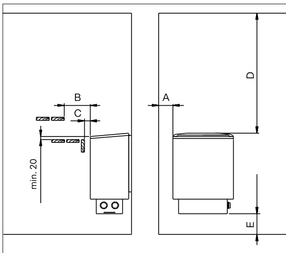
Kuva 1. Kiukaan suojaetäisyydet
