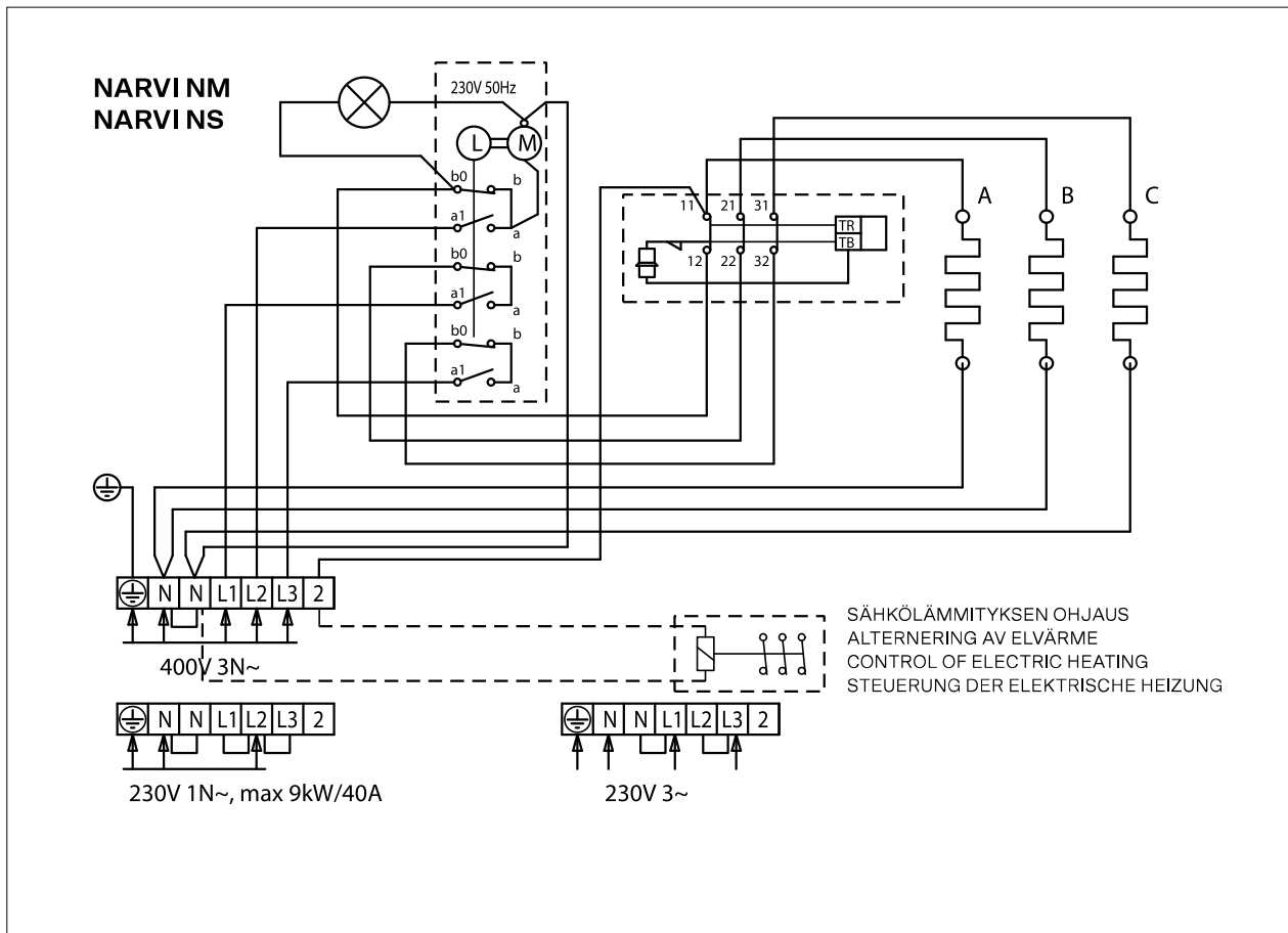
KytKentäkaavio
